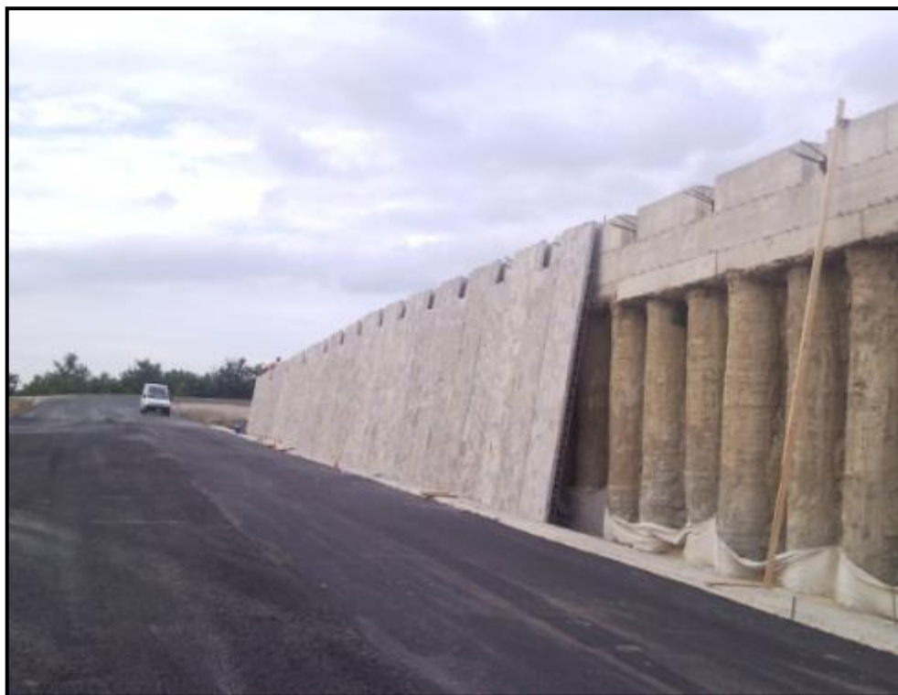
Figura 2 paratia rivestita - A.P.S. S.P. 73 località Frosini
